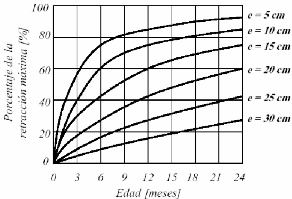
Figura N°5: Velocidad de retracción de losas de hormigón de diferentes espesores.
