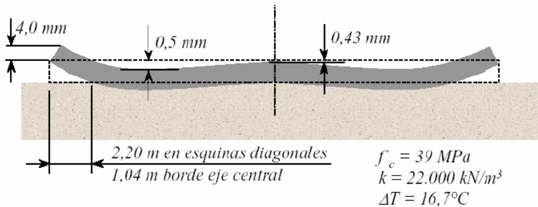
Figura N°2: Alabeo típico (fuera de escala) de una losa de hormigón de 15 cm de espesor apoyada sobre una base.
