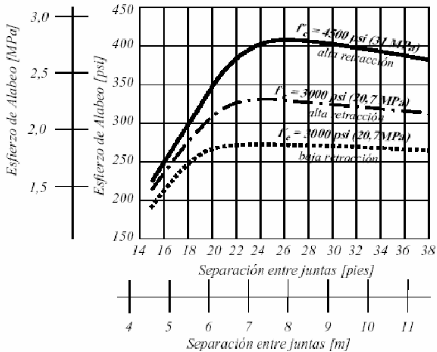
Figura N°4: Esfuerzo de alabeo generado en una losa de hormigón de 15 cm de espesor apoyada sobre una base con distintos niveles de resistencia y retracción del hormigón. Fuente: J. Holland & otros, 2001. "Seminario Internacional sobre Nuevas Tecnologías para Pisos Industriales". Park Hyatt Hotel, 24 y 25 de abril de 2001.
