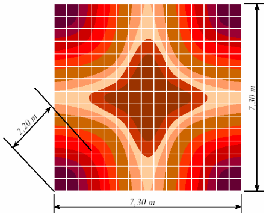
Figura N°3: Estado de tensiones de una losa de hormigón de 15 cm de espesor apoyada sobre una base.
